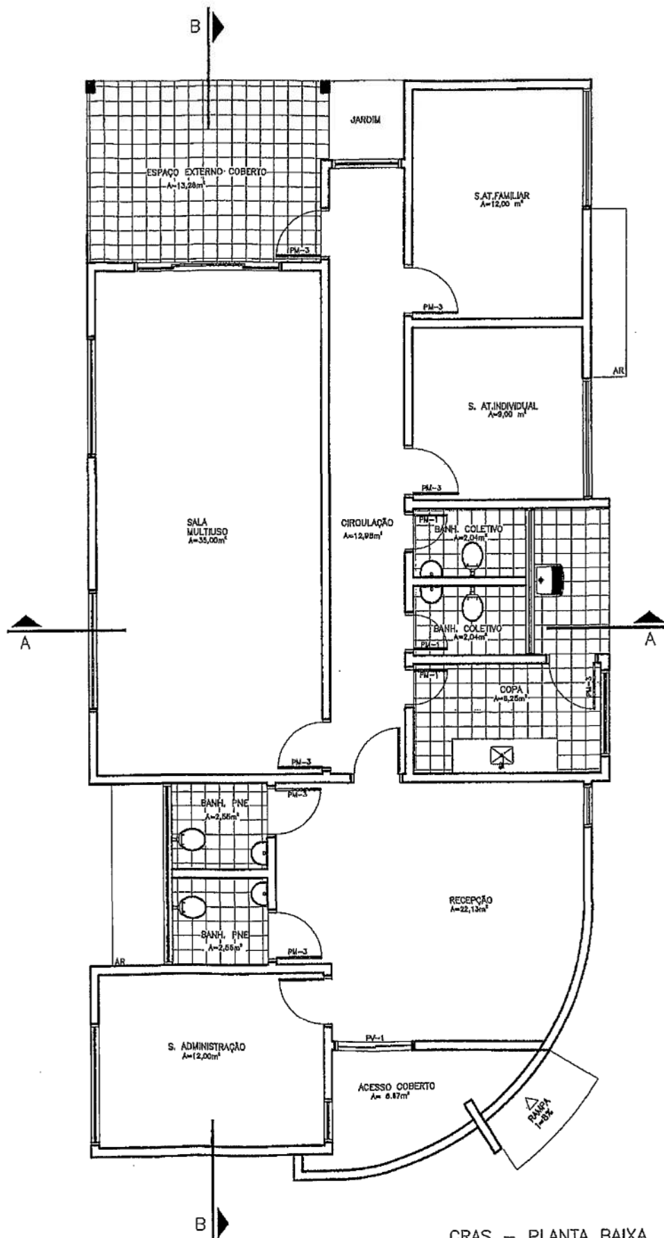
CRAS — PLANTA BAIXA ÁREA: 155,60 m²
