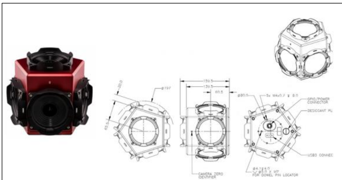
Figura 78 Modelo Câmera Ladybug com 6 câmeras acopladas
