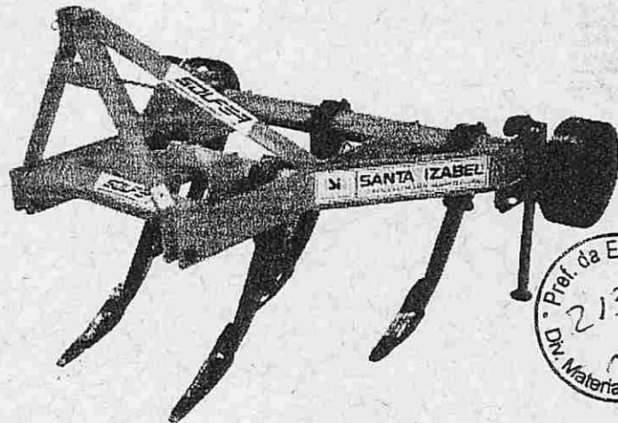
Subsolador com Desarme Automático Subsoiler Plow with Automatic Disarm Sobsolador con Desarme Automatico
