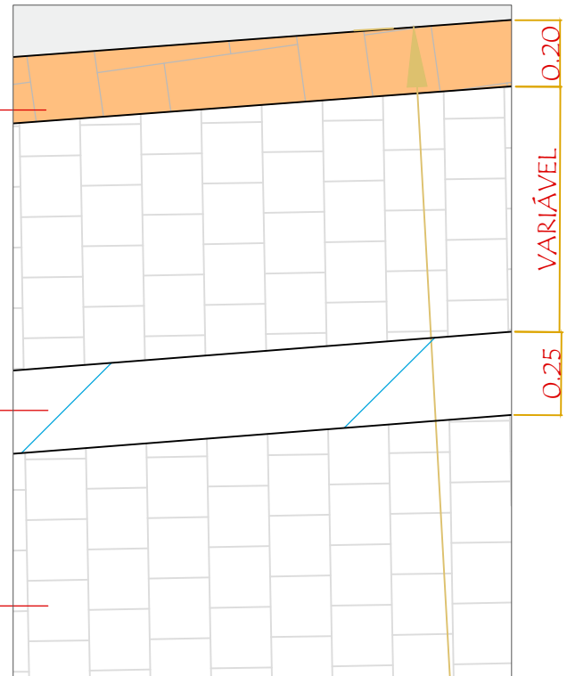
DETALHE 01 - PAGINAÇÃO DE PISO ESC: 1/100
