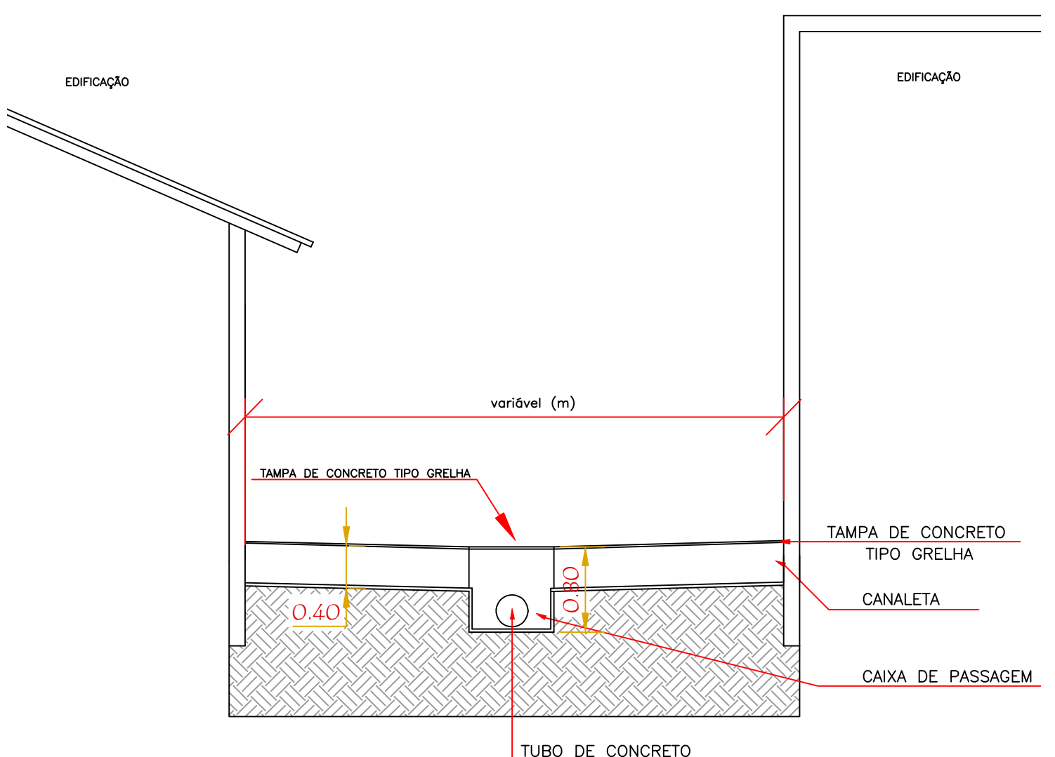
CORTE ESQUEMÁTICO SEM ESCALA
