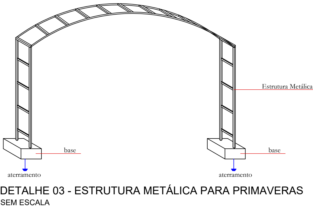
DETALHE 03 - ESTRUTURA METÁLICA PARA PRIMAVERAS SEM ESCALA
