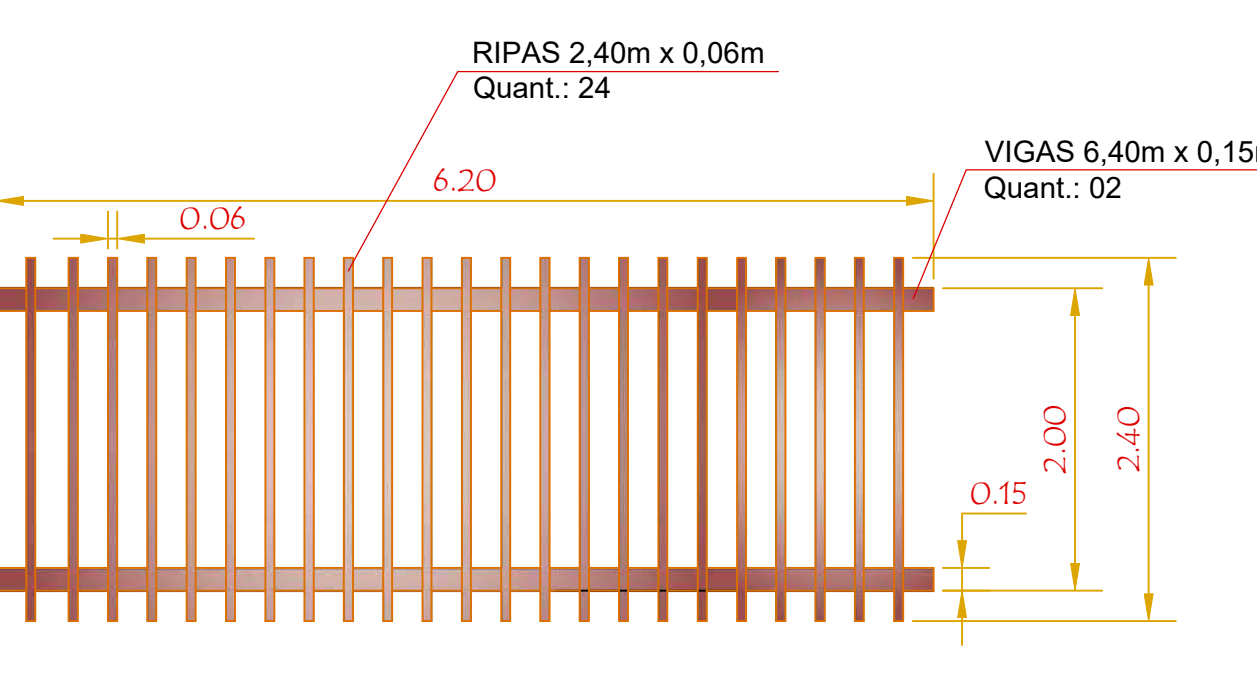
DETALHE 03 - PERGOLADO h=3,50m SEM ESCALA
