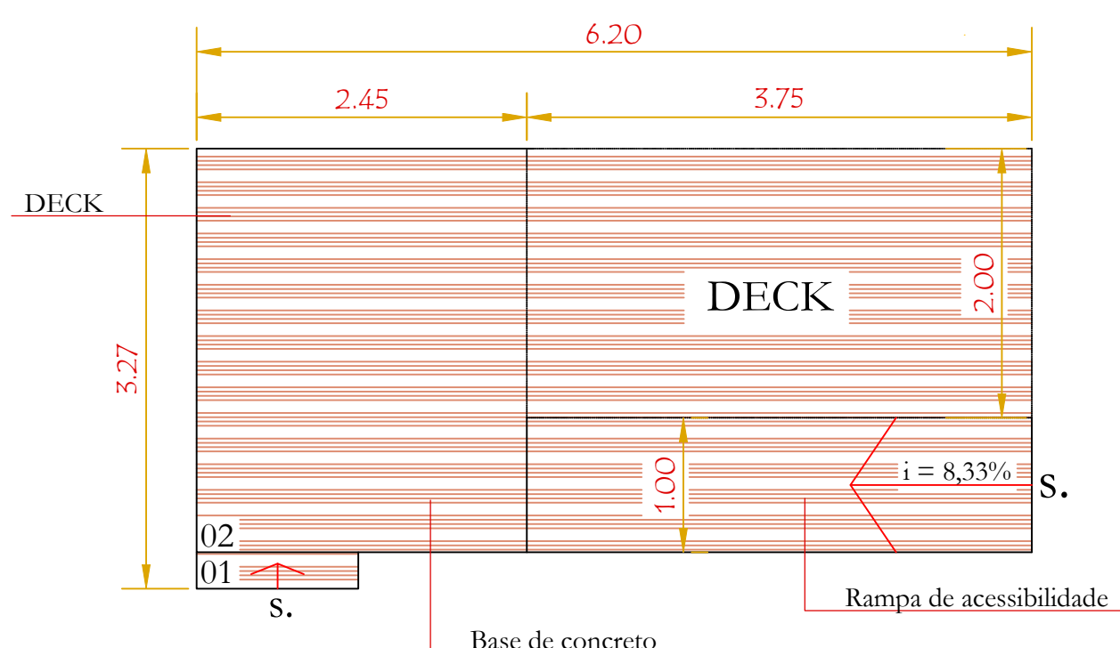
DETALHE 04 - DECK SEM ESCALA
