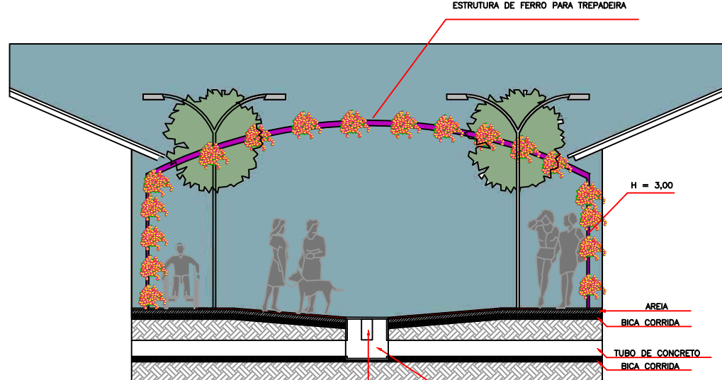
CORTE TRANSVERSAL TÍPICO DOS PLATÔS SEM ESCALA
