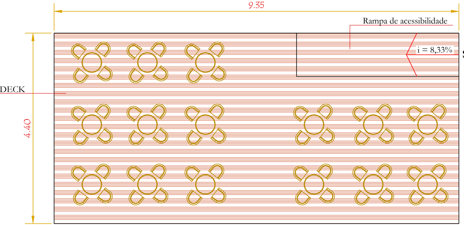
DETALHE 05 - DECK SEM ESCALA
