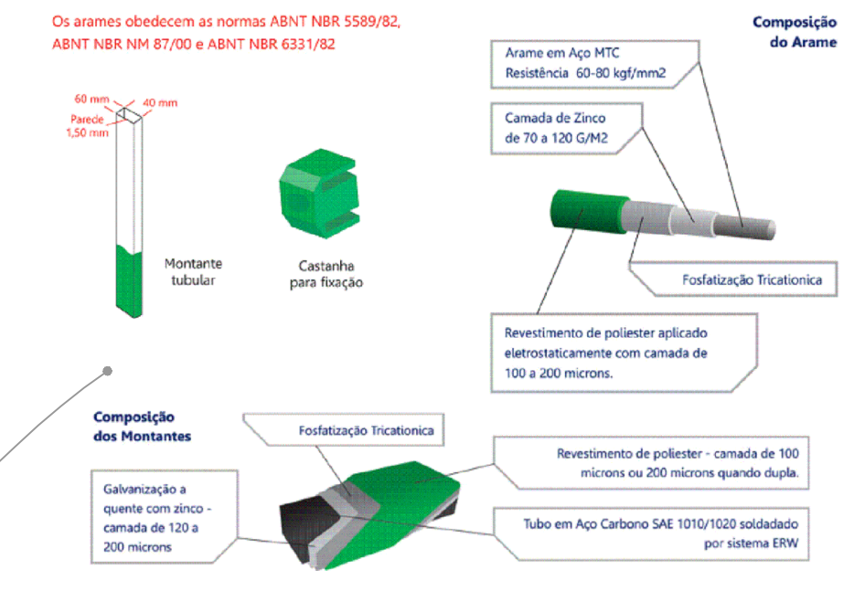
COMPONENTE - DETALHE 02
