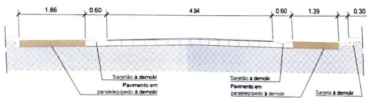
SEÇÃO TRANSVERSAL - AV. JOÃO PESSOA Escala 1:50
